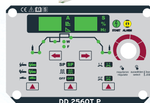
DD 2560T P vezérlőpanel
