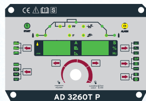
Vezérlőpult AD 3260T P
