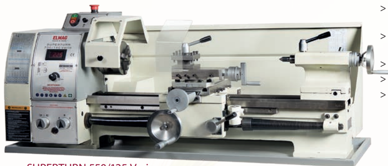
SUPERTURN 550/125 Vario
